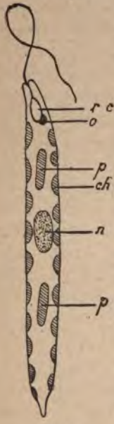
Fig. 4. Euglenadeses.
